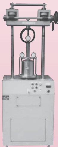
KS-60 CBR試験2本柱式載荷装置（力計別売り）
