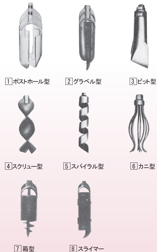
KS-97 ハンドオーガー刃先
