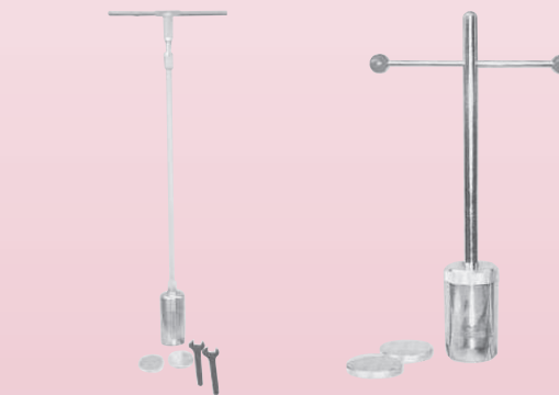
KS-98 円筒打込式サンプラー
