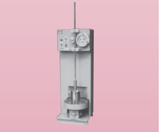
KS-55 土のオートランマー
