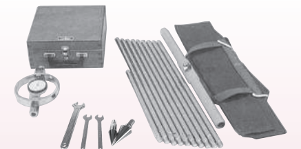
KS-159 コーンペネトロメーター
