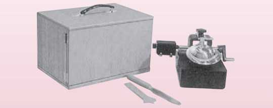
KS-39 カウンター付液性限界測定器
