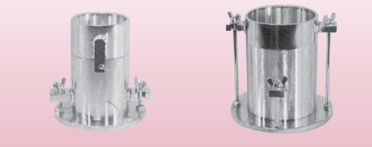
KS-44 10cmモールド
