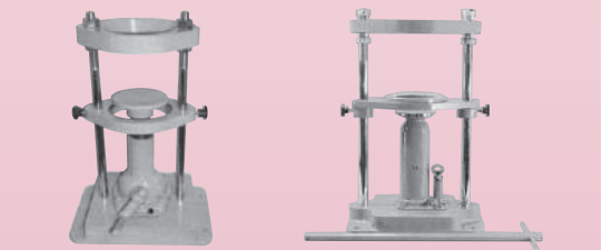
KS-50 A 試料採取器(スクリュージャッキ式)
