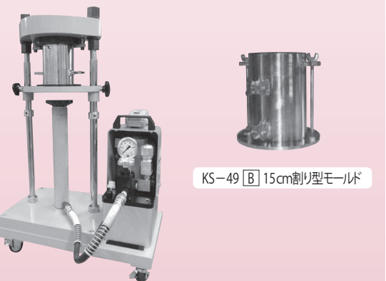
KS-206 電動式試料押出し機
