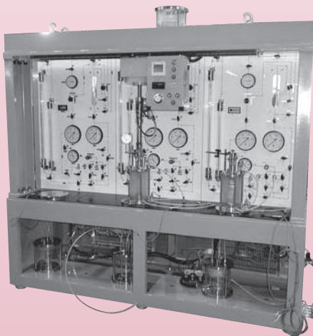
KS-214 三連型三軸試験装置
