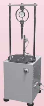
KS-212 コーン指数貫入装置
